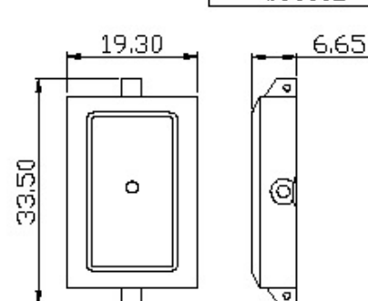
Mov't 2035 material: SS S9333L
