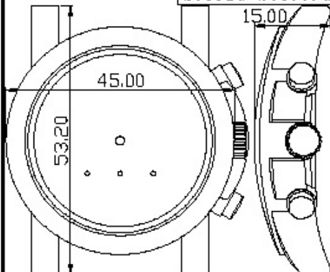
Mov't JS50 material: SS
