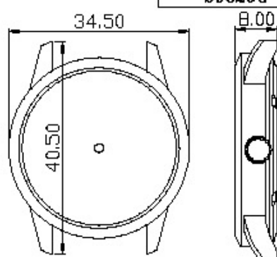
Mov't 2035 material: SS S9329G
